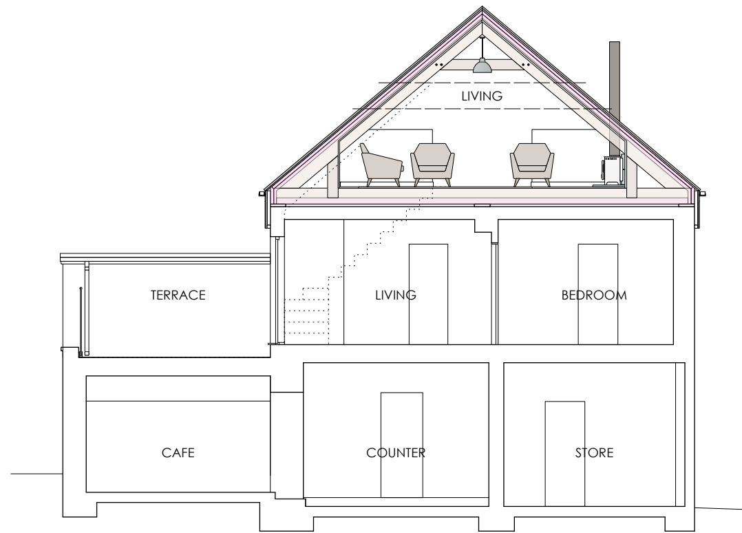
SECTION A-A
