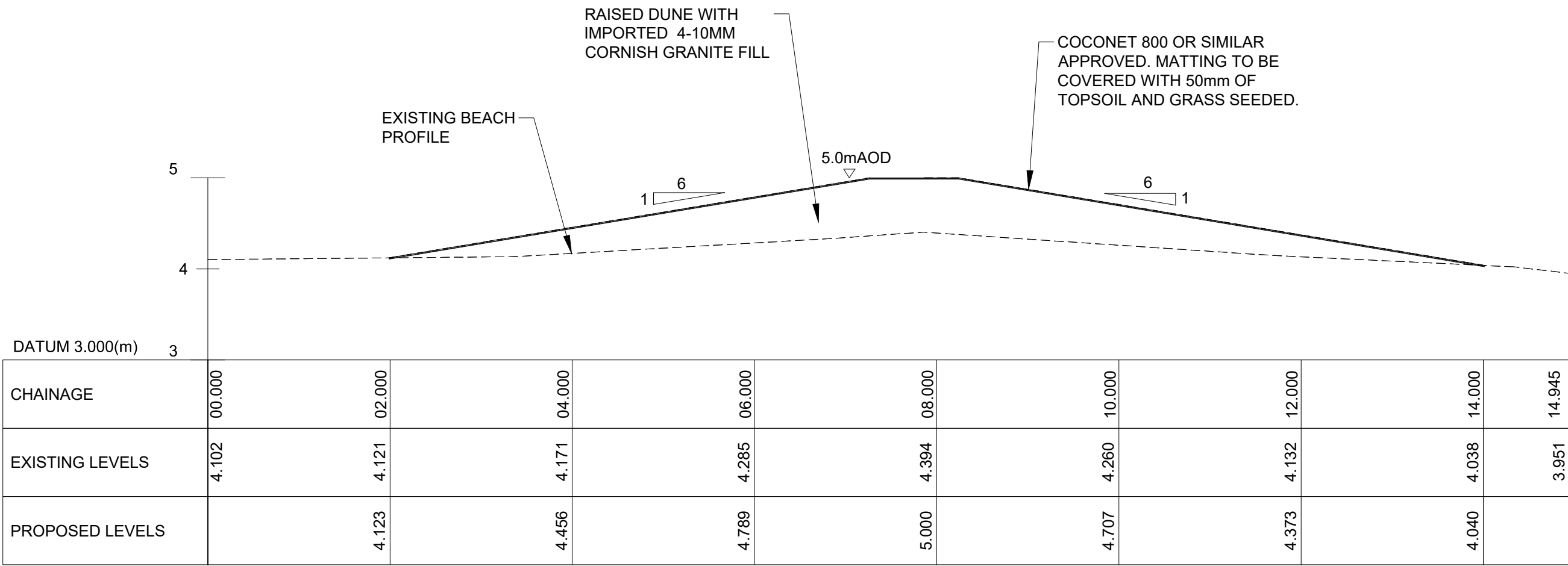
SECTION H 1 : 50
