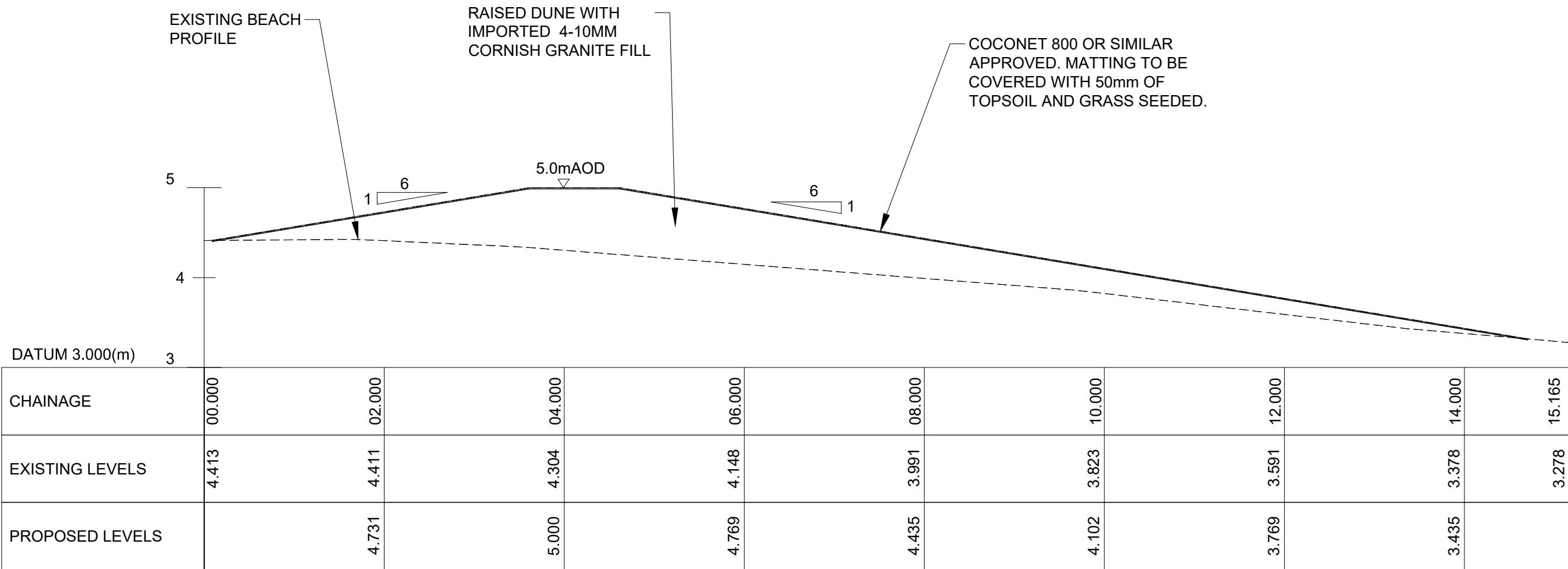
SECTION J 1 : 50
