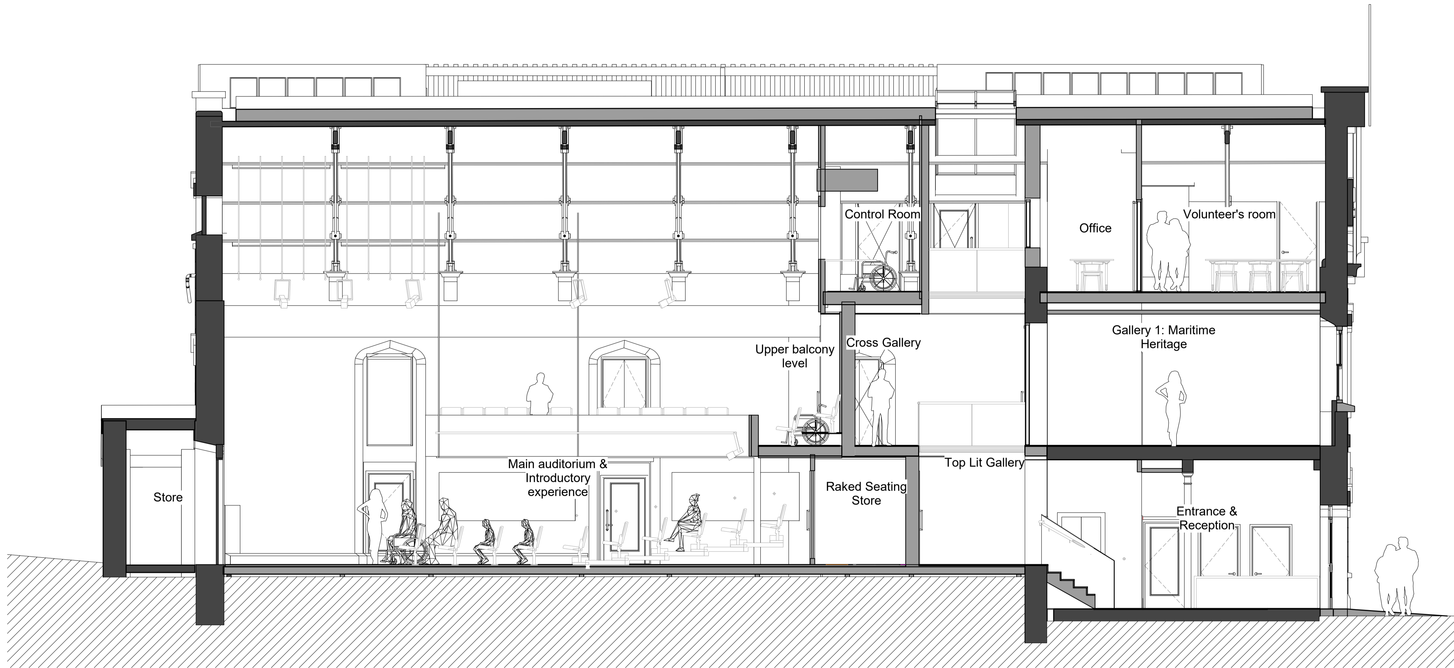
1 Section A-A 1 : 50
