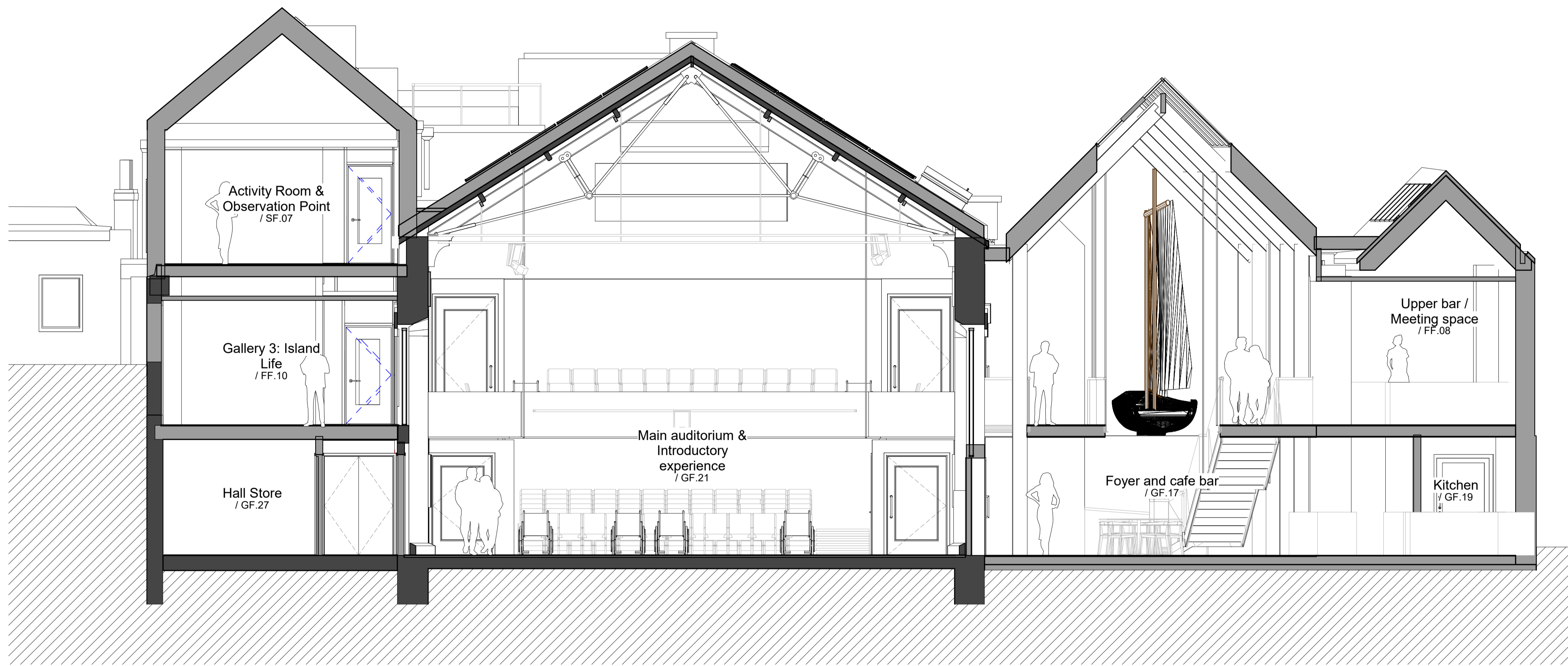
1 Section C-C 1 : 50
