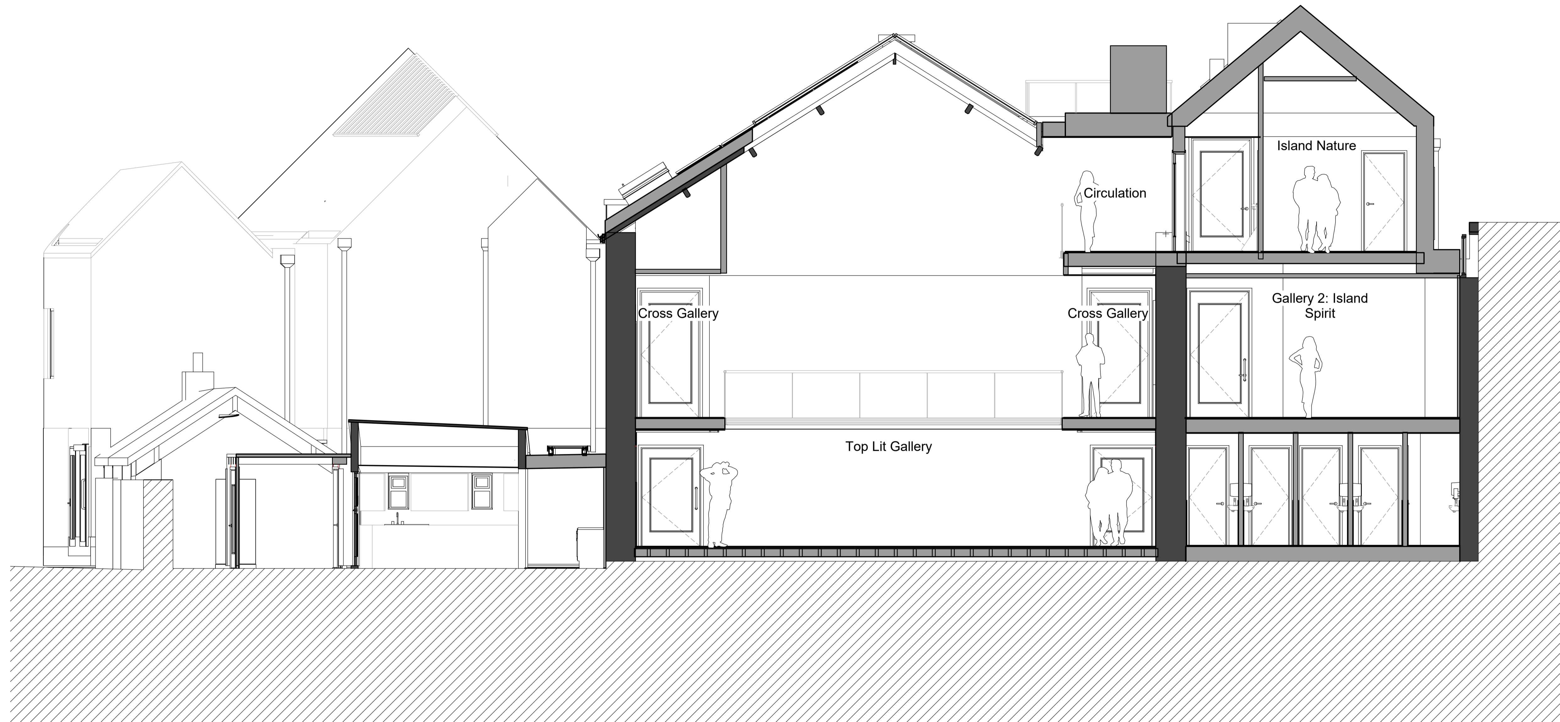
1 Section E-E 1 : 50
