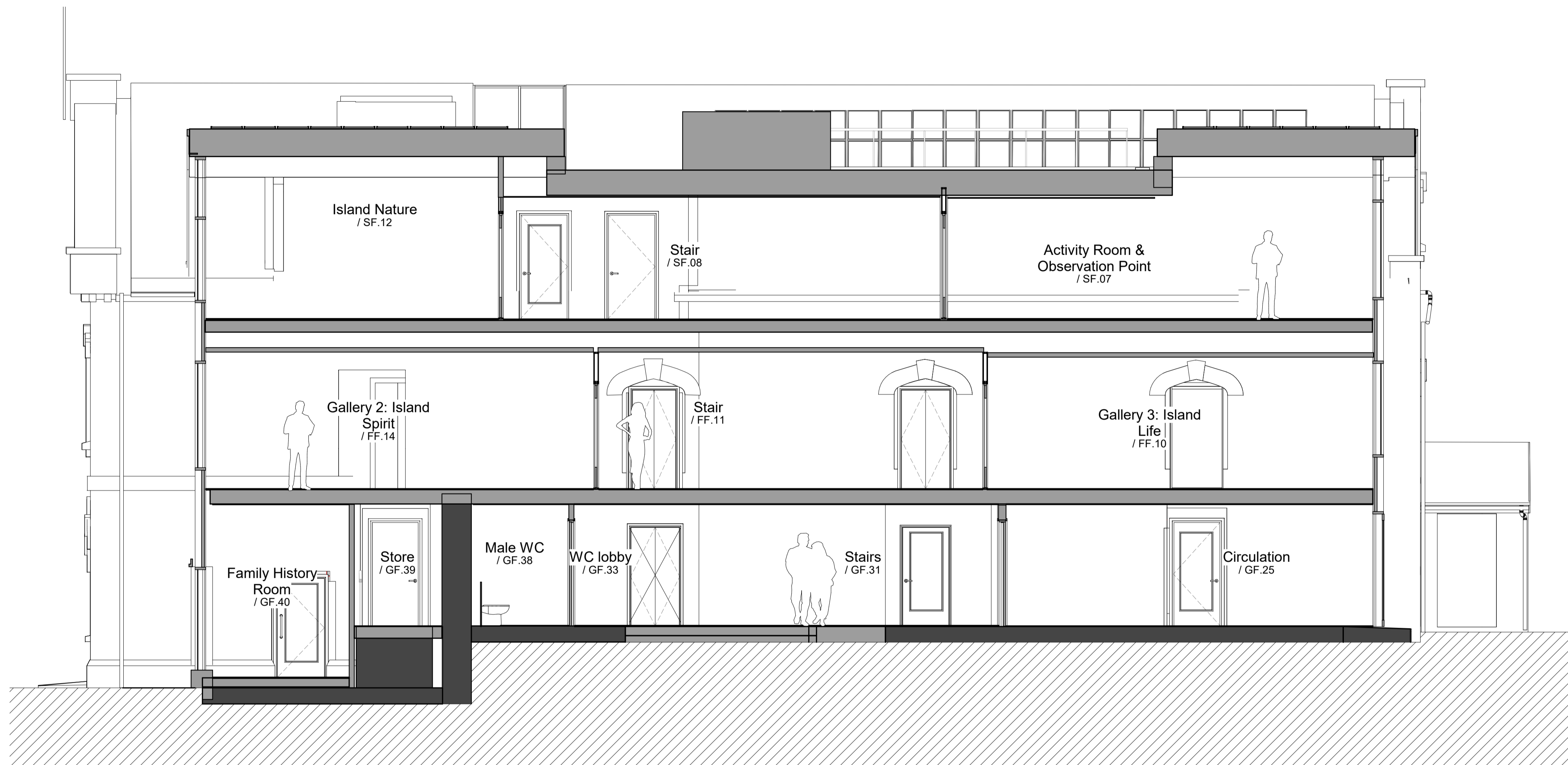
1 Section F-F 1 : 50
