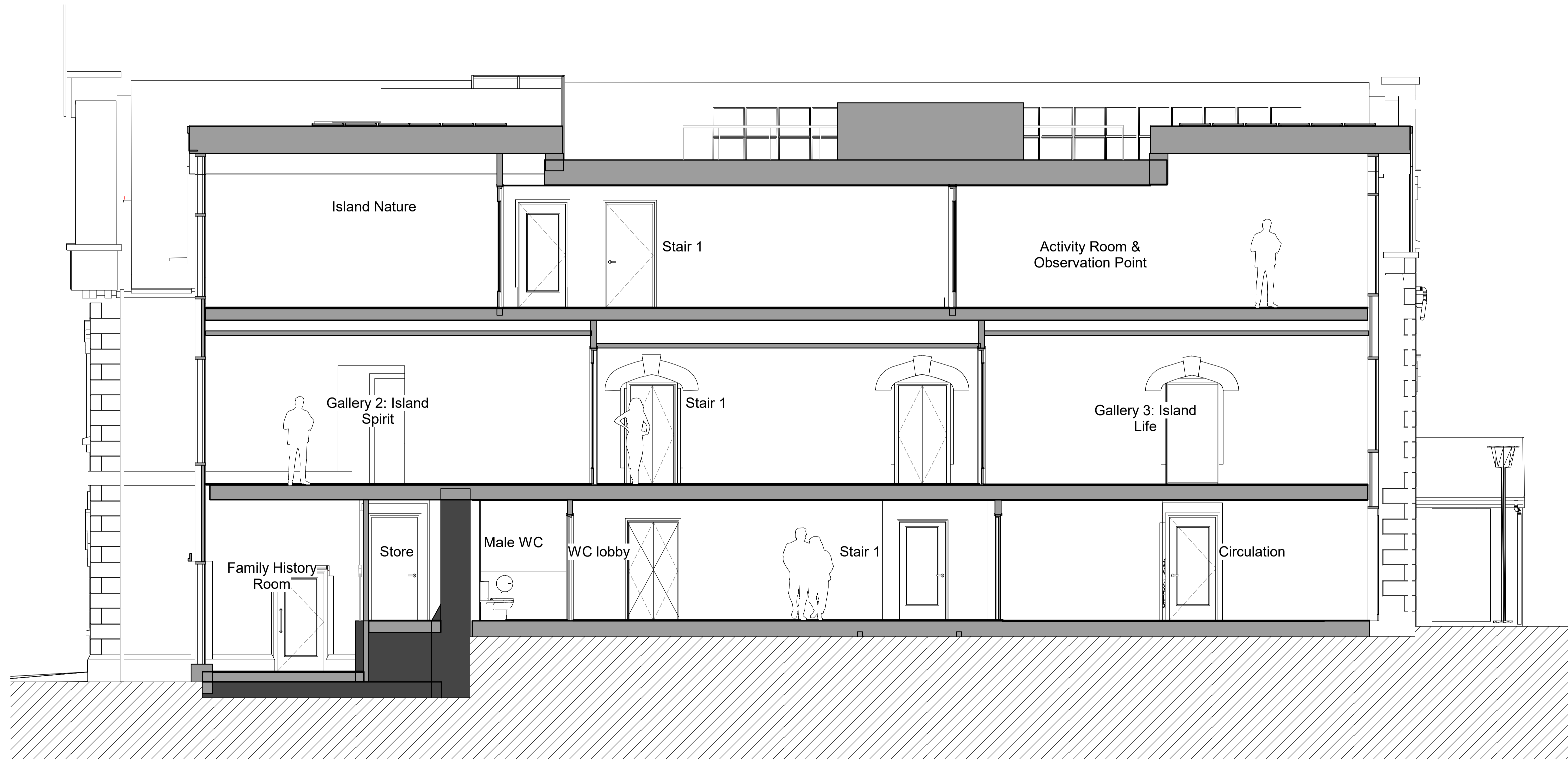
1 Section F-F 1 : 50
