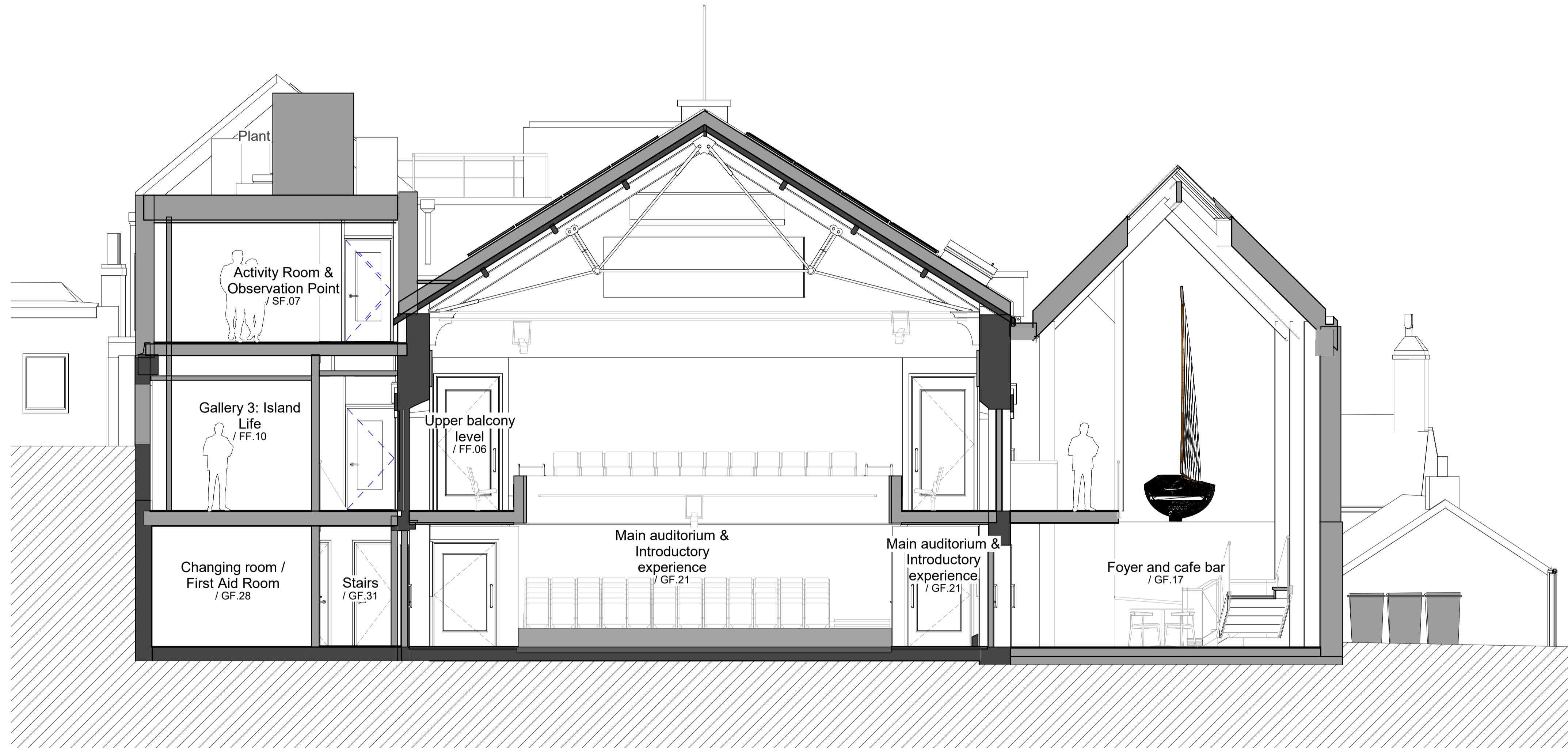
1 Section G-G 1 : 50
